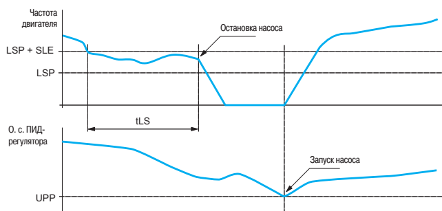
Функция ночного / дневного режима работы
