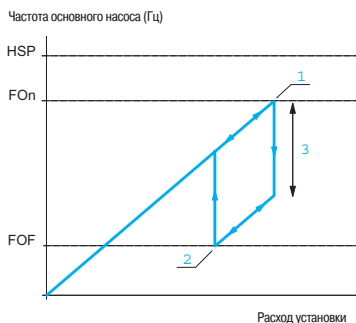
Работа основного и вспомогательного насосов: гистерезис
