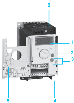
ПЧ ATV 12H075M2 с открытой передней крышкой
