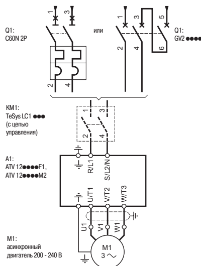
Управление двигателем при однофазном питании
