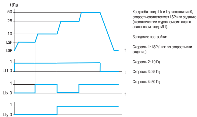
Пример работы с 4 заданными скоростями
