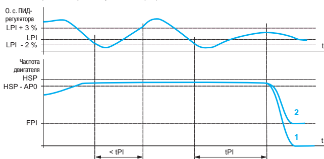
Контроль обратной связи ПИД-регулятора
