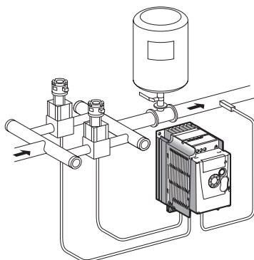
Режим работы основного и вспомогательного насосов
