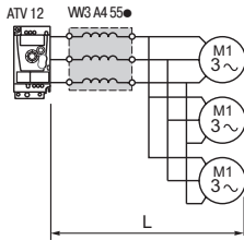
Сетевая дроссель
