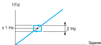
Пропуск частотного окна относительно резонансной точки
