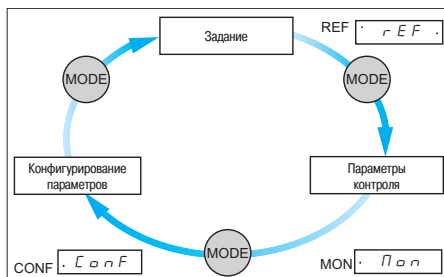
3 режима работы: REF, MON и CONF
