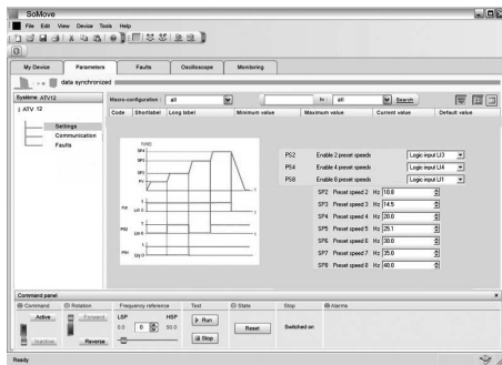
Настройка заданных скоростей с помощью ПО SoMove
