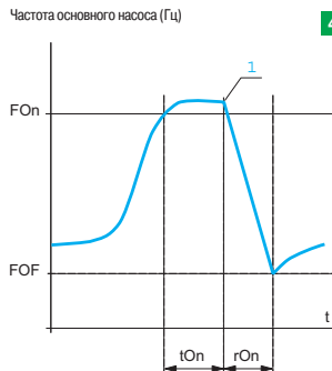
Пуск вспомогательного насоса
