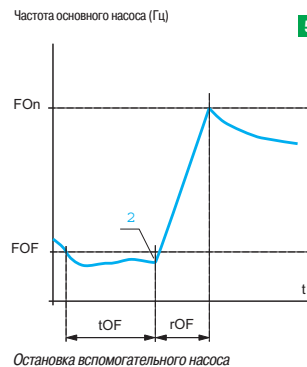
Остановка вспомогательного насоса
