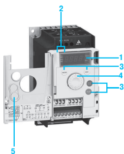
ATV 12H075M2 с открытой крышкой
