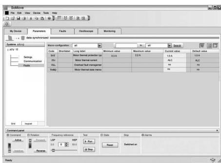
Настройка тепловой защиты с помощью ПО SoMove
