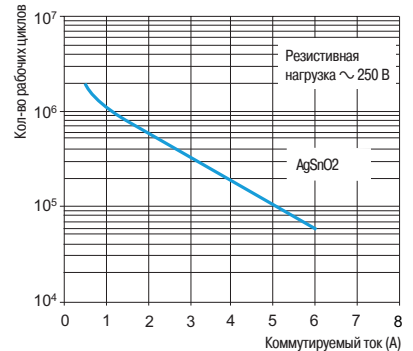
Электрическая износостойкость
