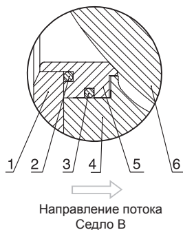
Металлическое седло
